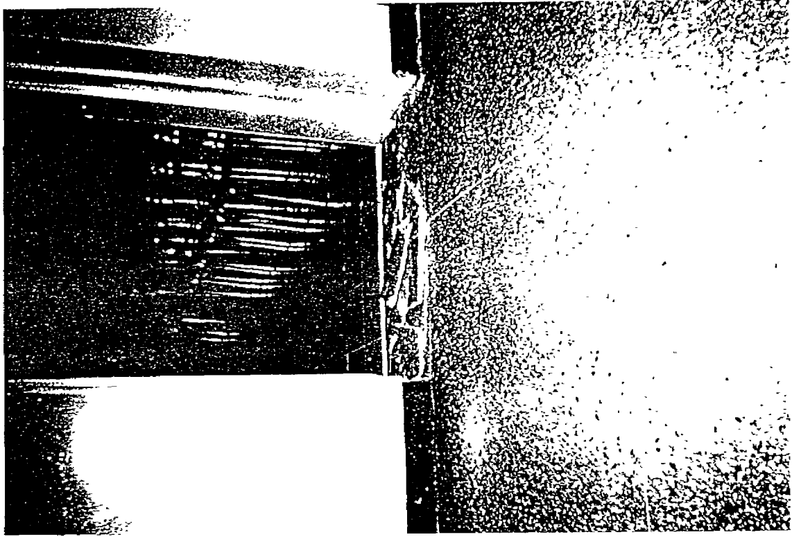
FOTO 2 ROTURA DE BALDOSAS POR ESTAR COLOCADAS EN LA JUNTA DE CONSTRUCCION HOSPITAL PATRICIO ALCALA
